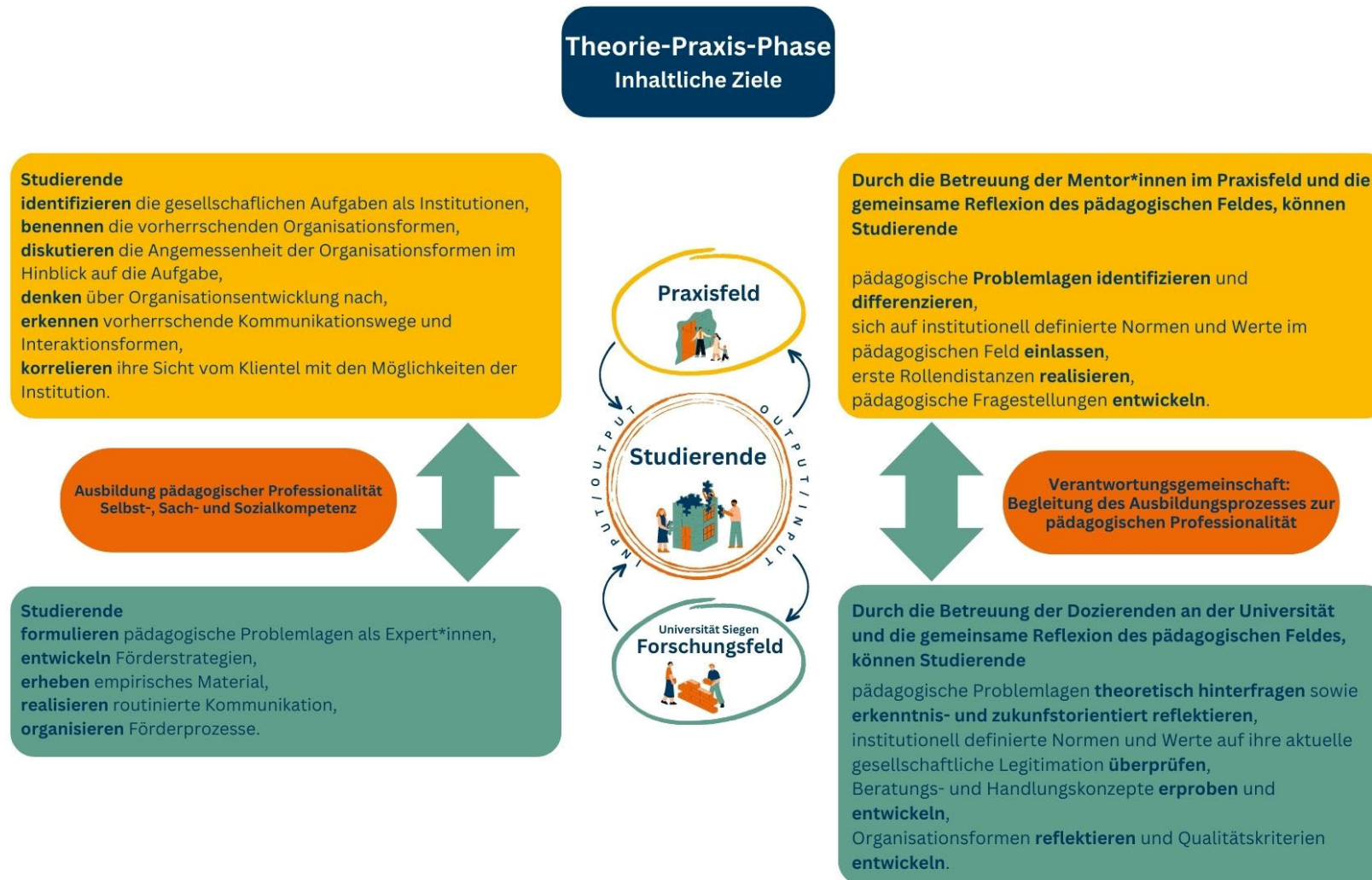
Abbildung 1: Korrelationsmodell Theorie-Praxis-Kopplung
